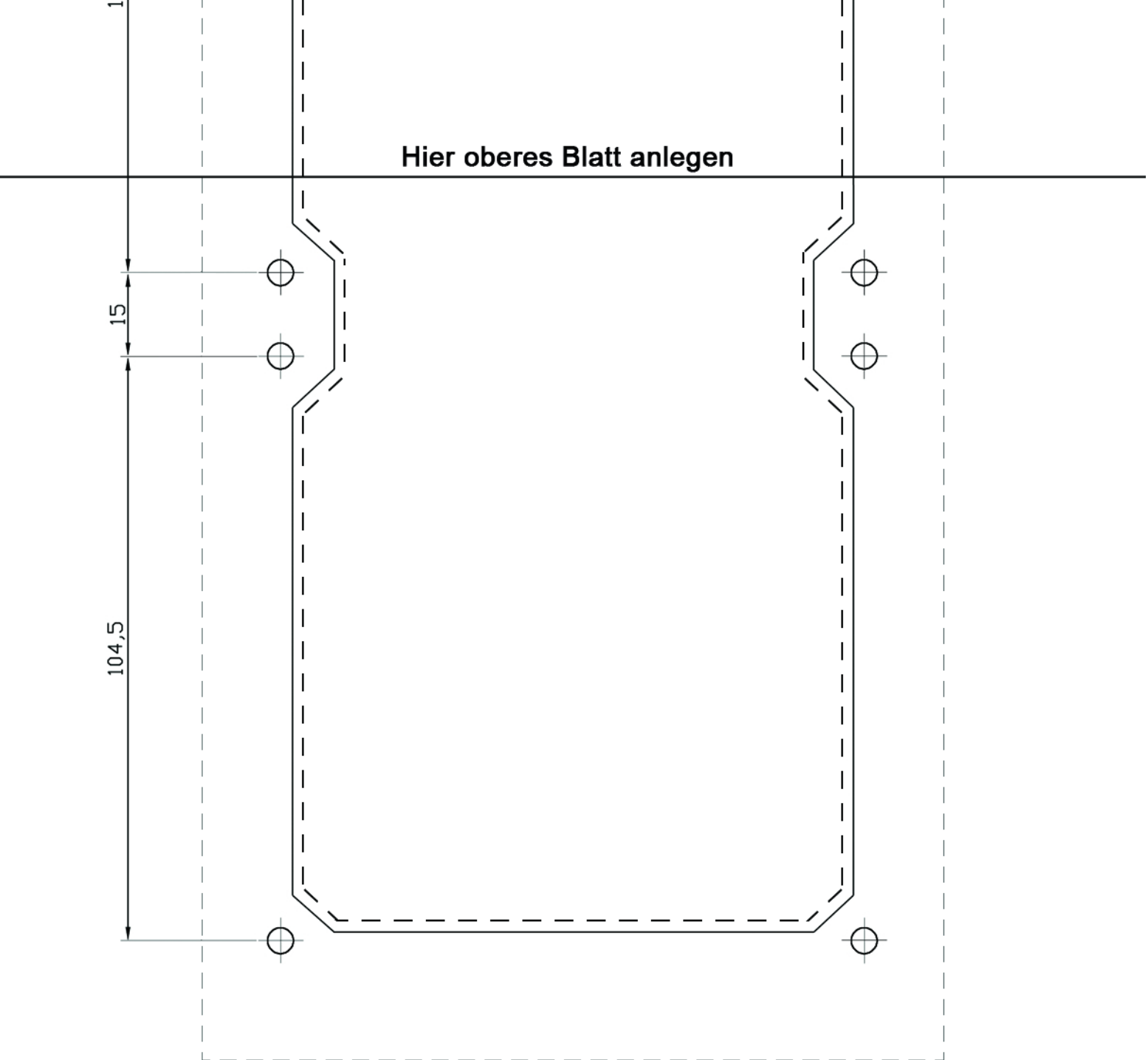
Einbauschablone Triple-Radiator
